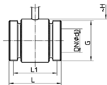
Sanitary connection per DIN 11851
